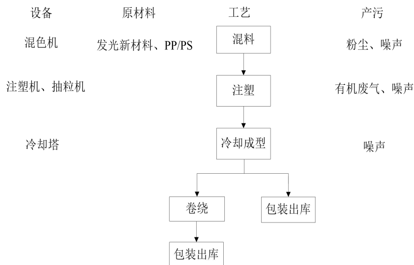
图 2-2 新型 3D 打印材料、新型发光制品生产工艺及产污环节图
